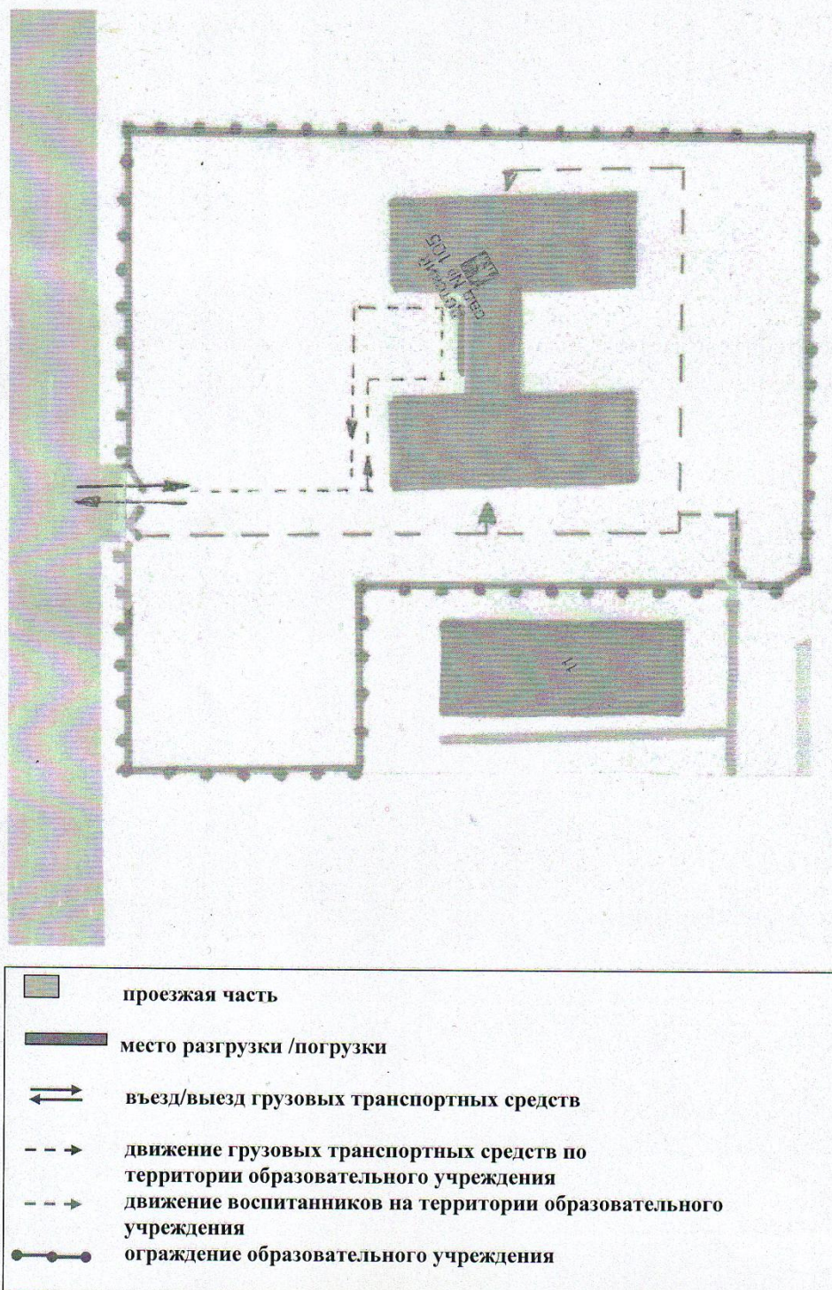
1.3. План – схема путей движения транспортных средств к местам разгрузки/погрузки и рекомендуемых безопасных путей передвижения воспитанников их родителей (или законных представителей) по территории ОУ
